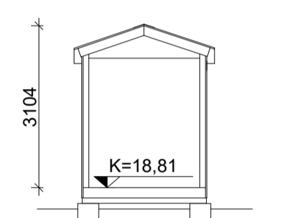
Snið í Tækjaskýli Tals Snið D 1 = 100 mm
