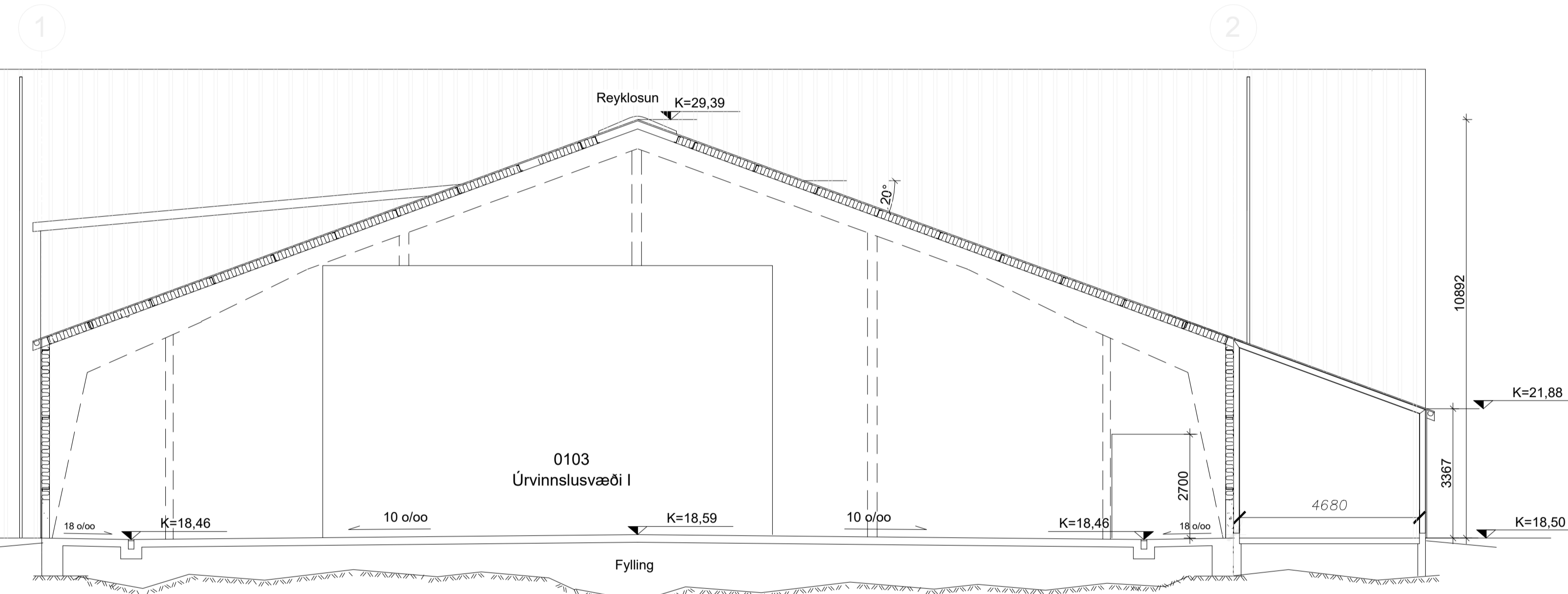
Snið B 1 = 100 mm
