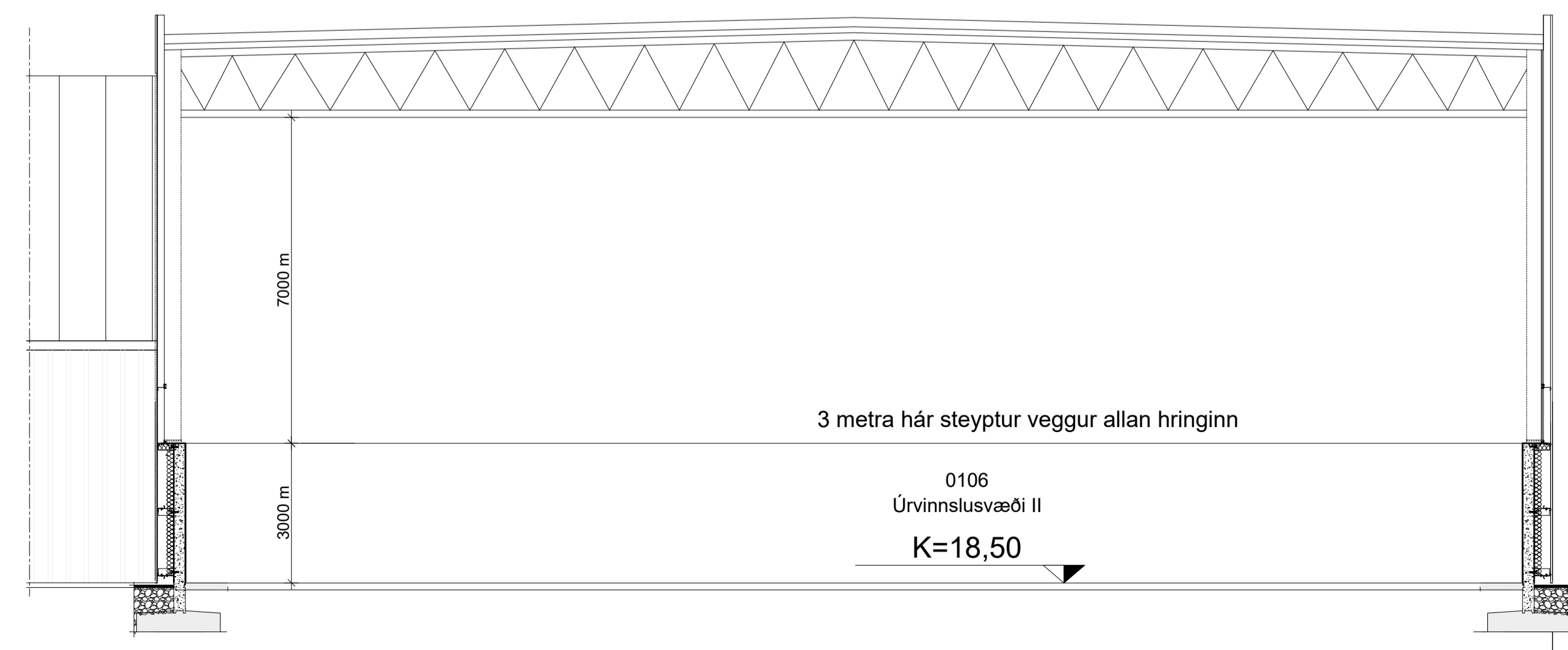
Snið E 1 = 100 mm
