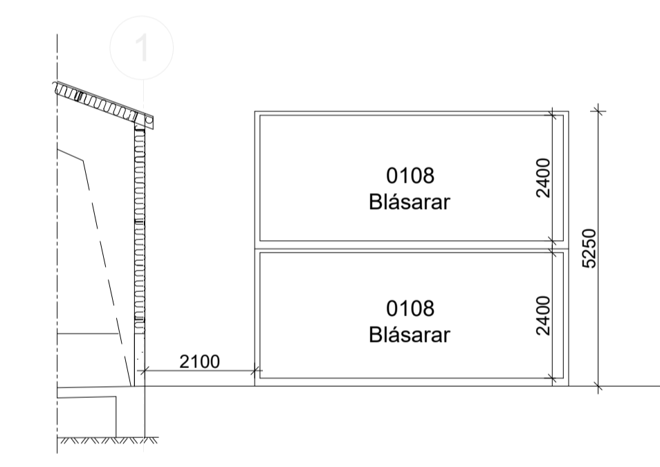
Snið F 1 = 100 mm
