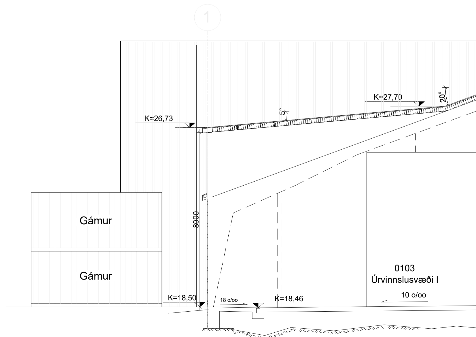
Snið C 1 = 100 mm
